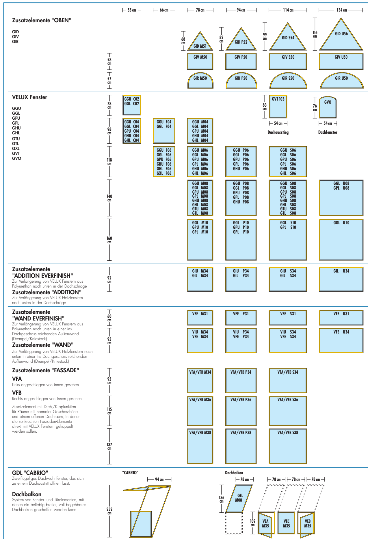
2 Dieses Raster gibt Ihnen eine Übersicht zu den Standardgrößen, damit Sie den Einbau von VELUX Dachwohnfenstern problemlos planen können.
